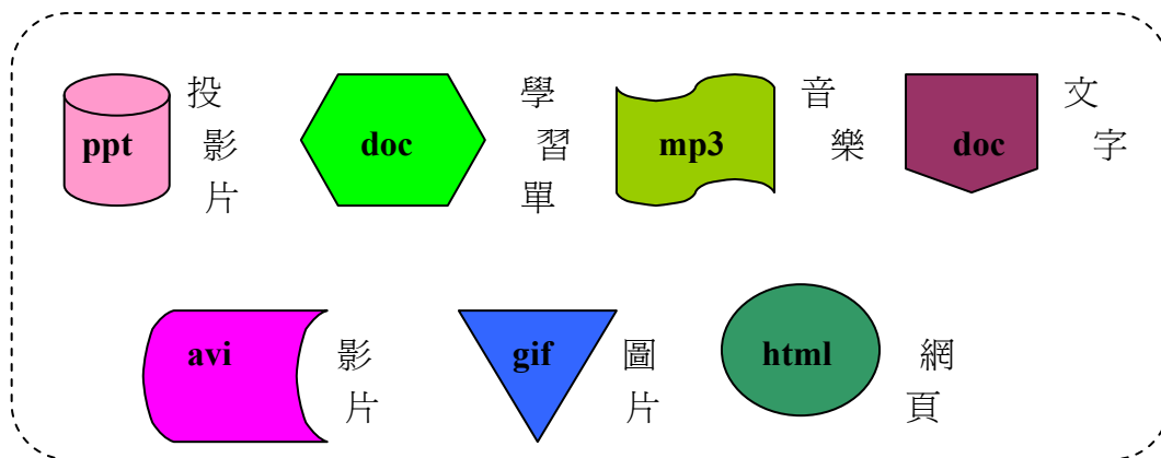
圖 4-3 素材示意圖
