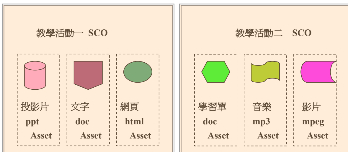
圖 4-4 SCO 示意圖
